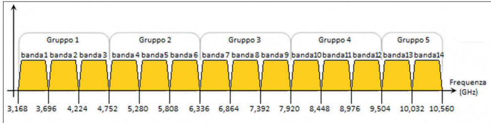
Figura A.14: Bande di frequenza per un sistema Multi-Band OFDM.
