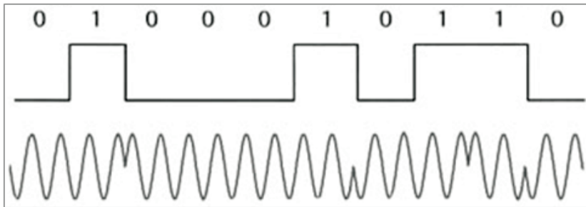
Figura 10: Modulazione PSK.
