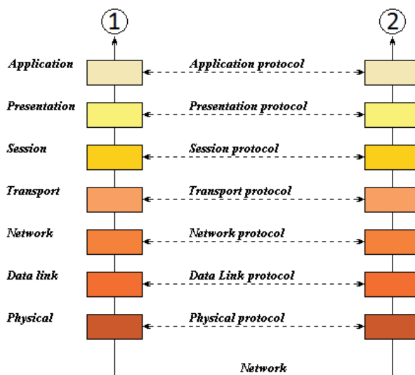
Figura 7: Modello OSI.
