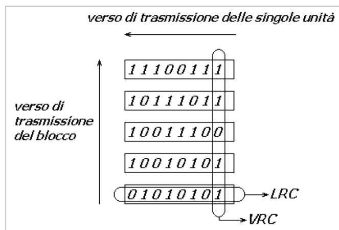
Figura 22: Algoritmo LRC.
